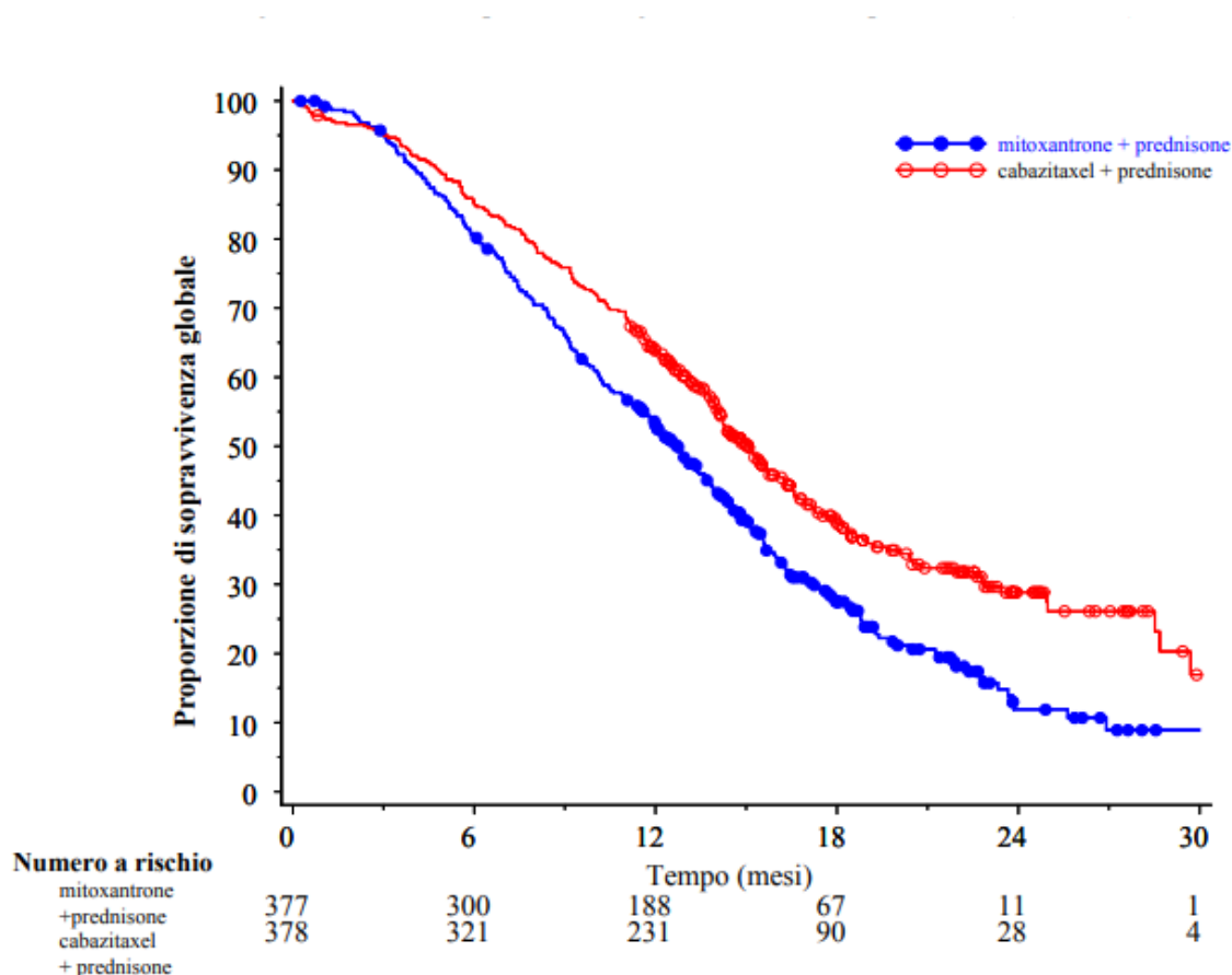
Figura 1: Curve di sopravvivenza globale secondo Kaplan Meier (EFC6193)
